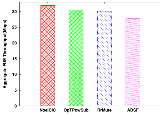
Figure 3.4: Aggregate FUE Throughput
